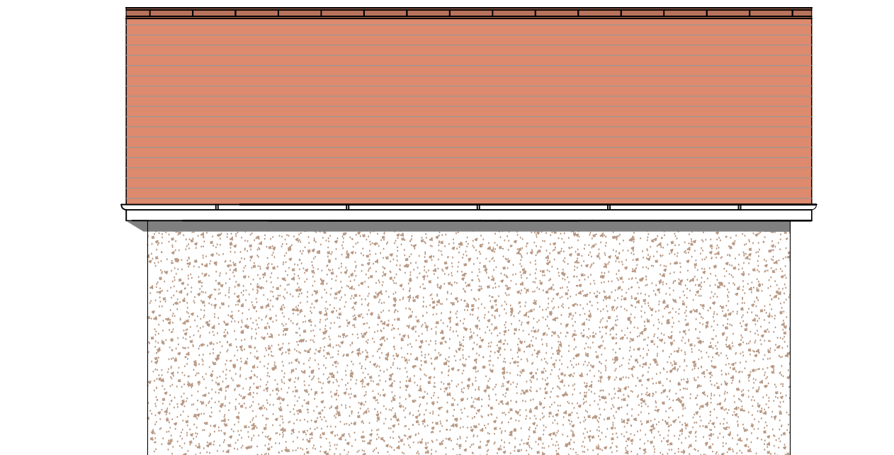
4 Elevation C & D 1:50
