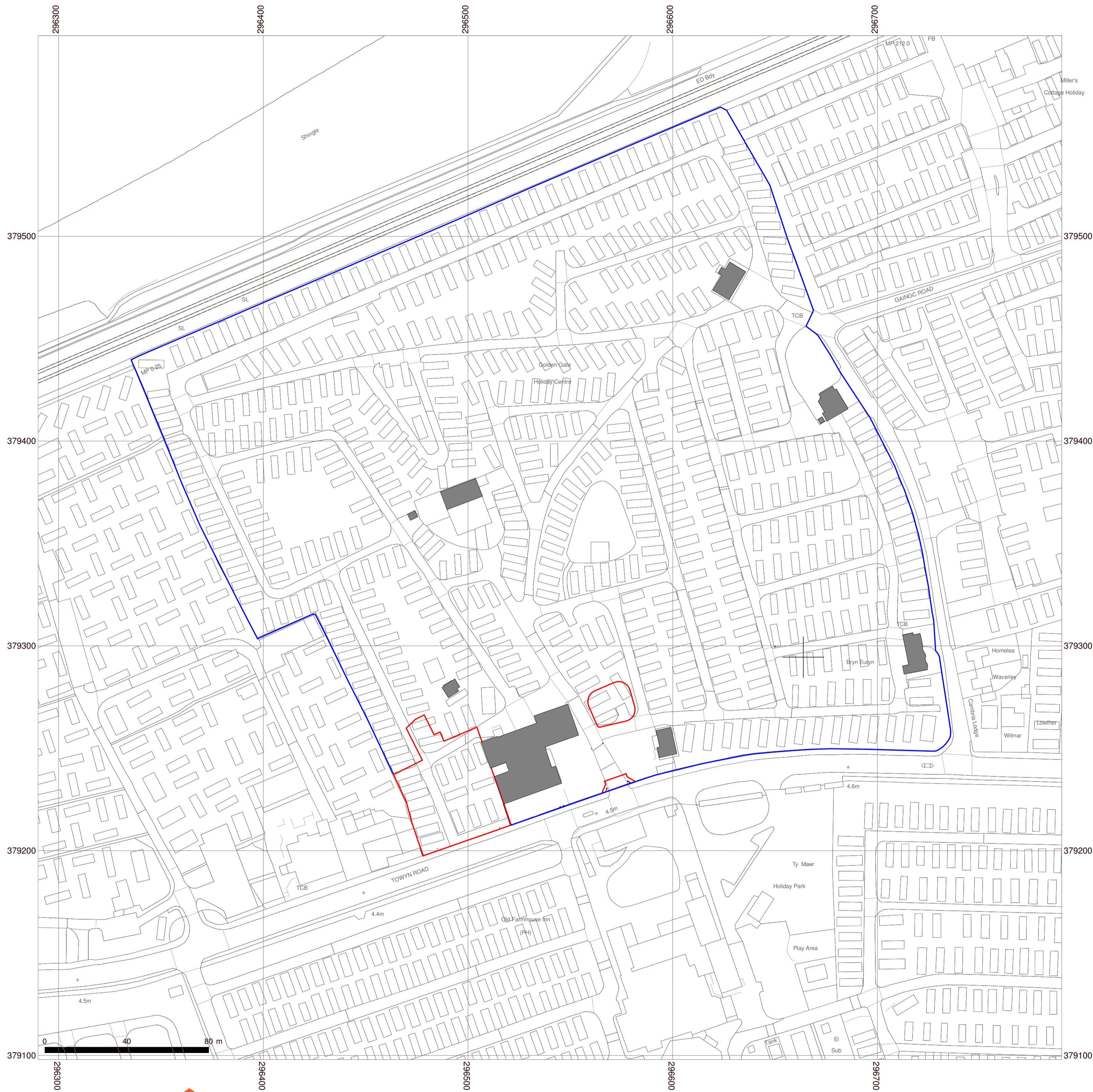
1 Site_Location_Plan Scale: 1 : 1250
